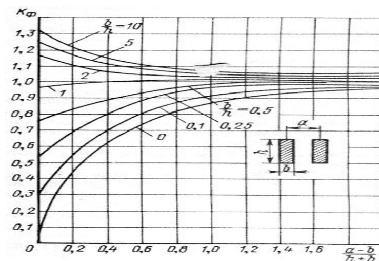
Рисунок 1 – Кривые для определения коэффициента формы K_{\phi}
